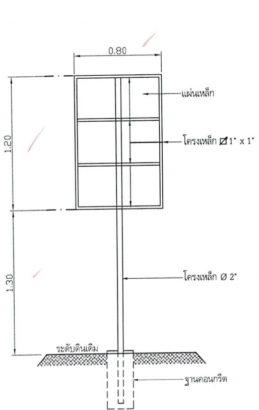
รูปด้านหลัง NOSCALE
