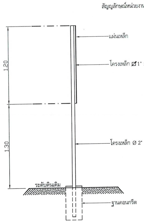
รูปด้านข้าง NOSCALE
