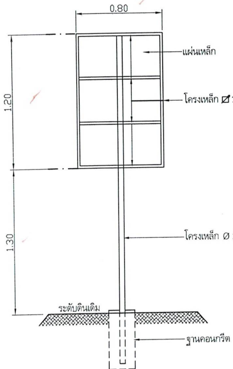
รูปด้านหลัง NOSCALE
